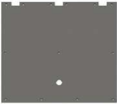
CNH-84981654 PLACA DESLIZANTE 610 X 550
