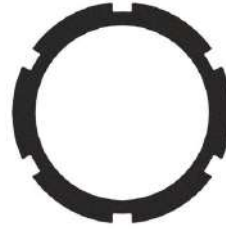
SC-15 ANEL INTERNO DISCO C/ 6 ENCAIXE 140 X 110 X 2MM
