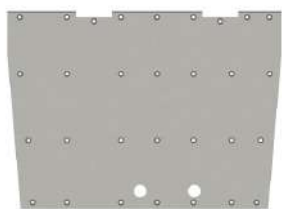
MF-6211872 PLACA DESLIZANTE 658 X 480
